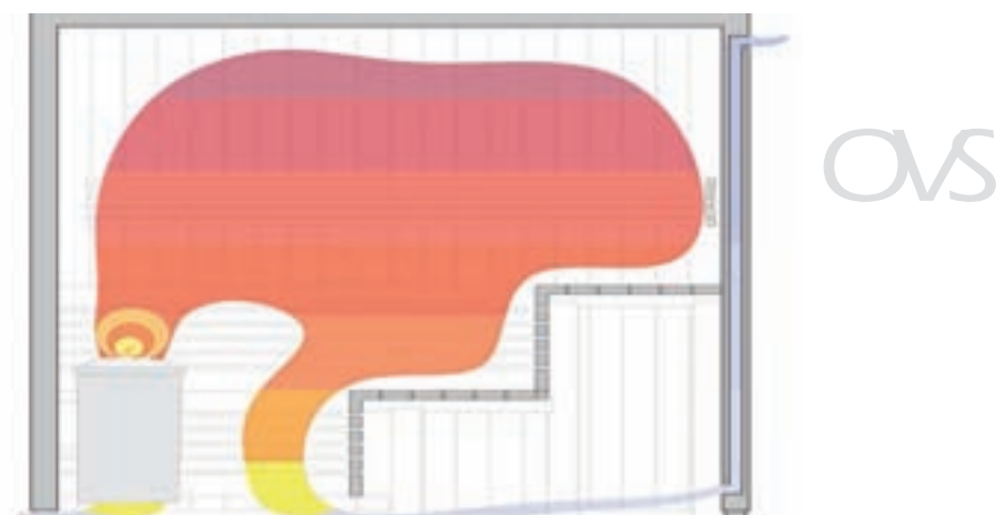
OVS Bonacina - Luft- und Wärmezirkulation in der Saunakabine
