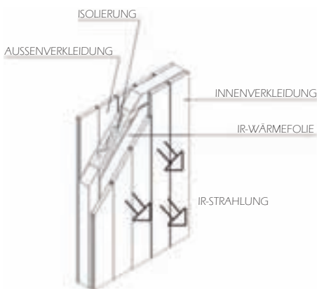
Einbau-Detail Infrarotfolien
